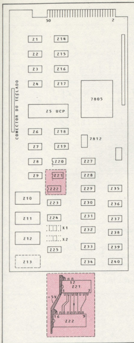
Figura 2 - Placa da UCP do D-8000 vista pelo lado de cima; observe no destaque feito embaixo que o corte no ponto "X" só será necessário quando do uso de uma quarta ROM no soquete Z13.
